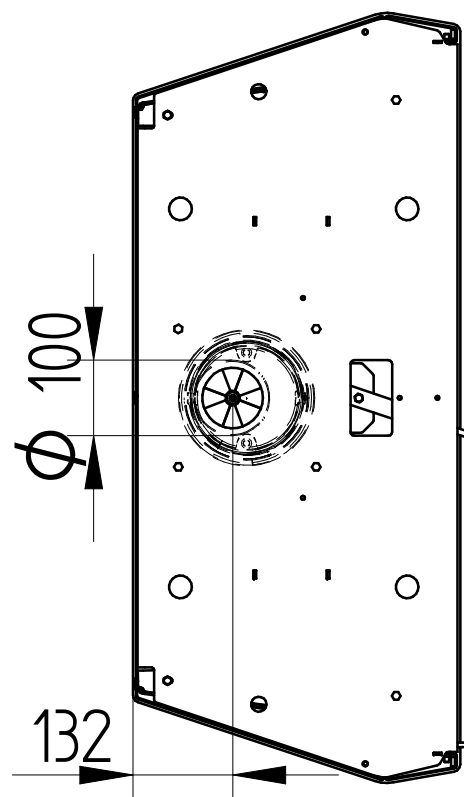
SECTION A-A
